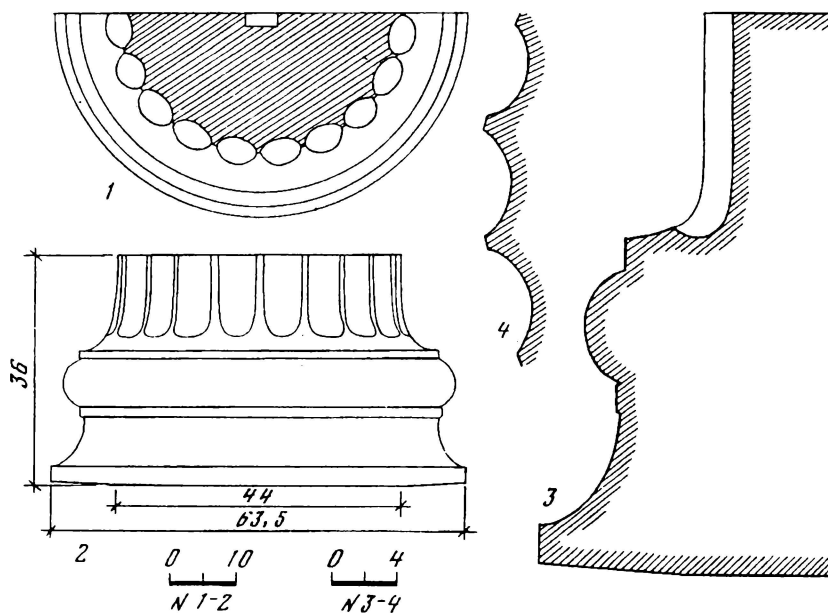
Рис. 11. Архитектурный обмер баз колонн
